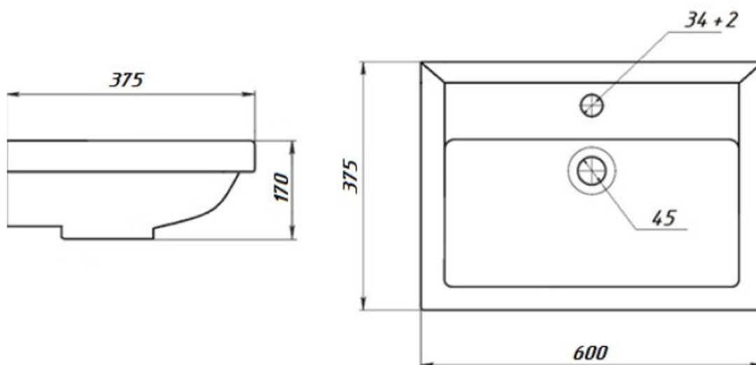
Чертёж умывальника
